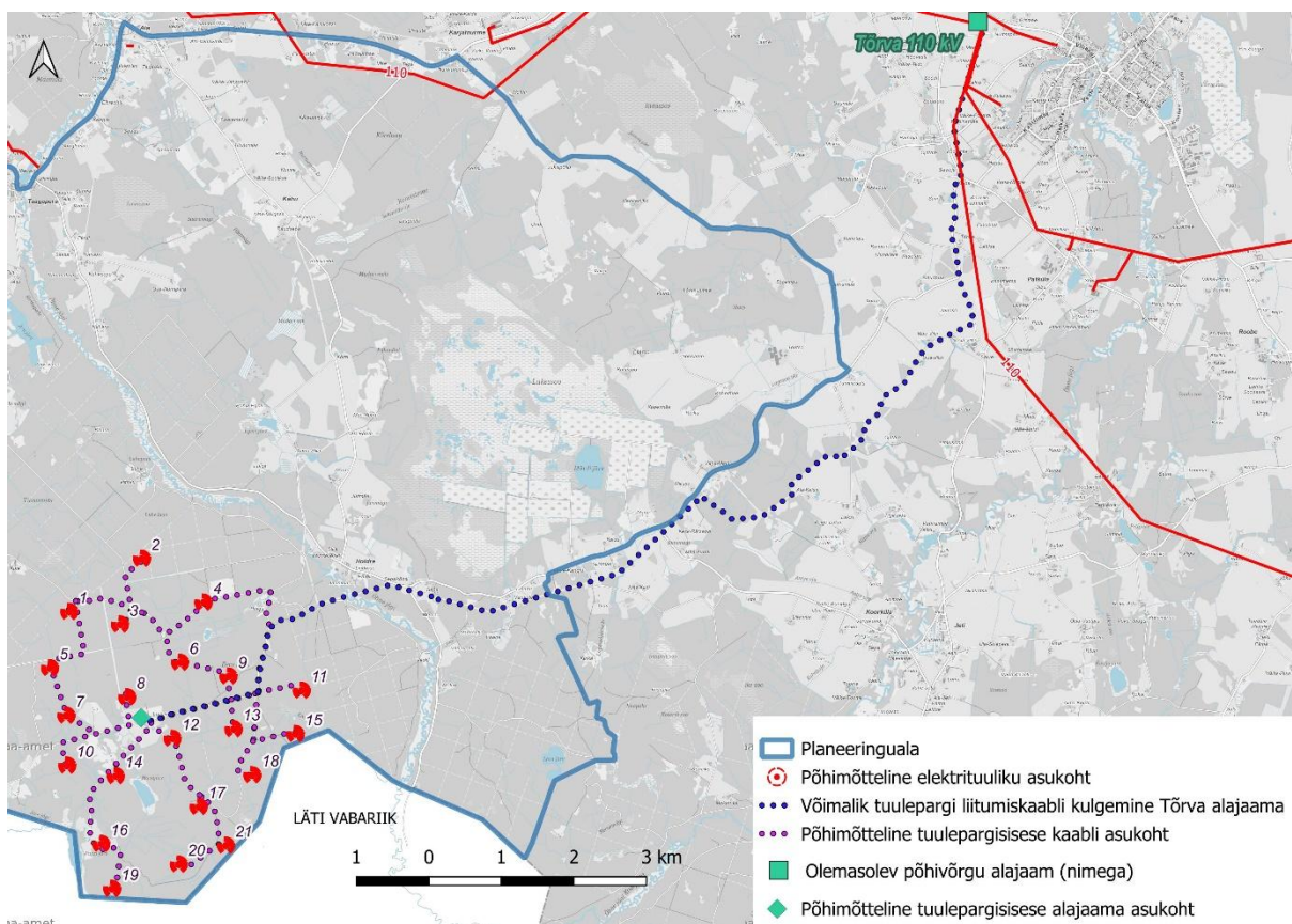
Joonis 5. Planeeritud tuuleparki teenindavate maakaabelliinide põhimõtteline paiknemine.
